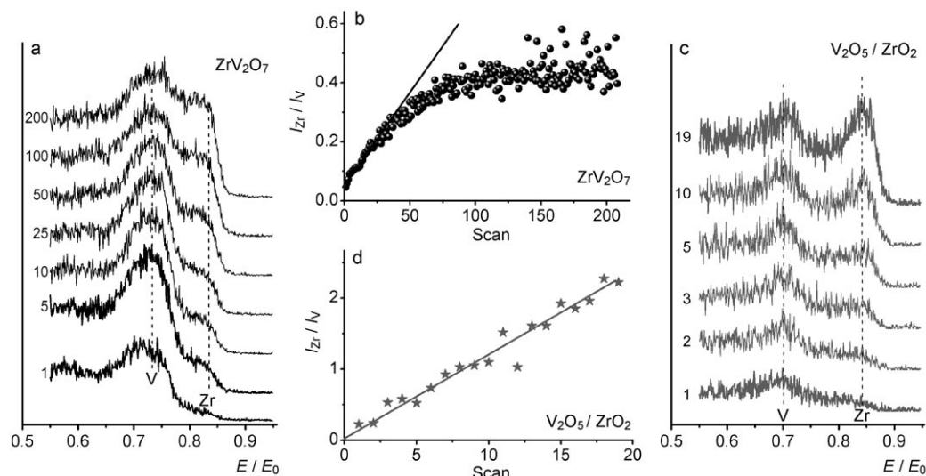
Abbildung 1. LEIS-Sputterserien und Intensitätstrends von Zr-V-Mischoxiden ( E_0 = 1000 eV). a, b) \text{ZrV}_2\text{O}_7 , c, d) 4 Gew.-% \text{V}_2\text{O}_5 auf \text{ZrO}_2 (V-Gehalt (7.5 Atome pro \text{nm}^2 ) nahe der theoretischen Monolagenkapazität, vgl. Tabelle S1).
