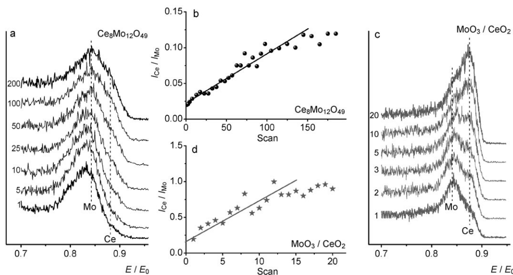
Abbildung 2. LEIS-Sputterserien und Intensitätstrends von Ce-Mo-Mischoxiden. a, b) \text{Ce}_8\text{Mo}_{12}\text{O}_{49} , E_0 = 1000 eV, c, d) 2.7 Gew.-% \text{MoO}_3 auf \text{CeO}_2 (Mo-Gehalt (3.6 Atome pro \text{nm}^2 ) ca. 80% der theoretischen Monolagenkapazität, vgl. Tabelle S1), E_0 = 2000 eV.
